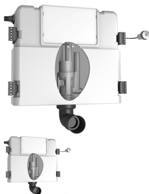
Réservoir WC à déclenchement sans contact manuel
