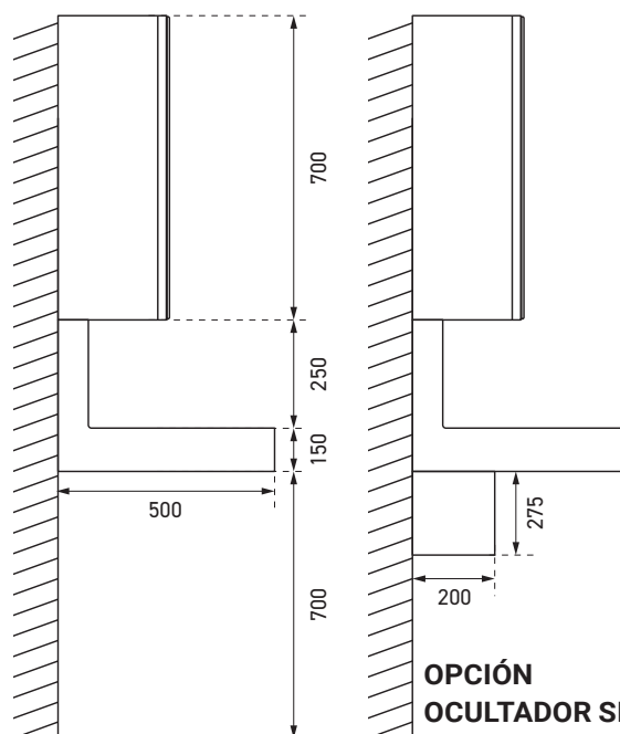
Lavabo material compuesto para modulo espejo L600 x A395 x P495 mm REF. LA-600
