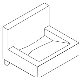
Lavabo material compuesto para módulo espejo L600 x A395 x P495 mm REF. LA-600
