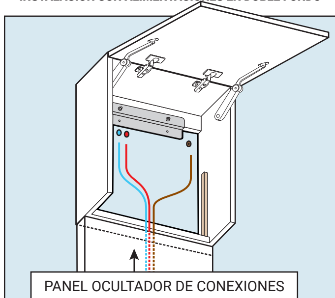
INSTALACIÓN CON ALIMENTACIONES EN DOBLE FONDO
