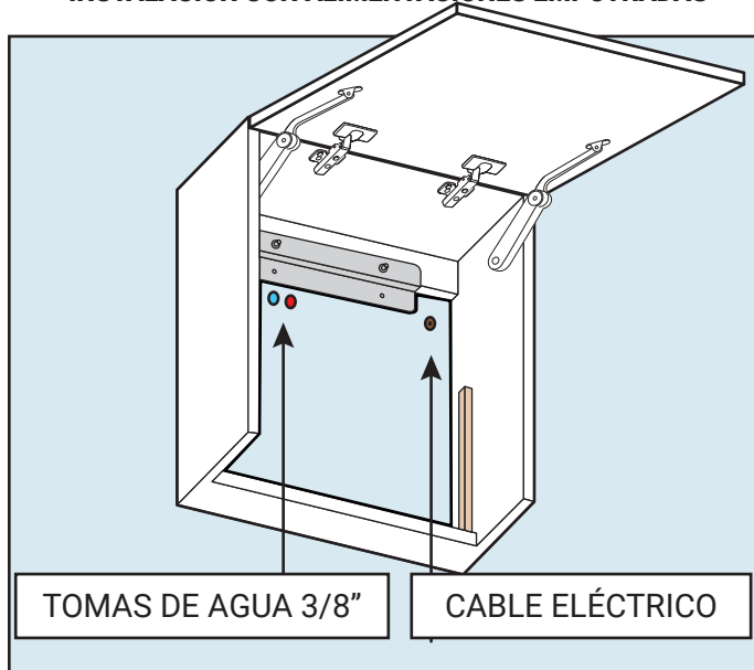
INSTALACIÓN CON ALIMENTACIONES EMPOTRADAS
