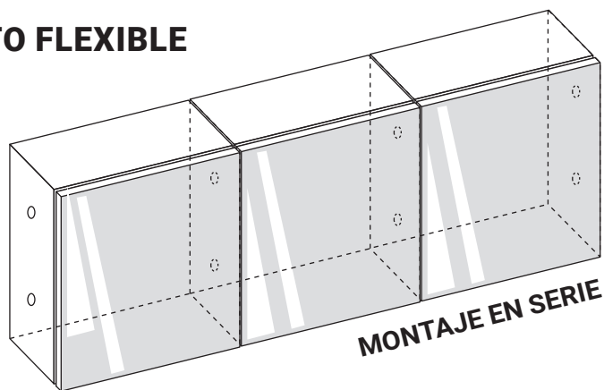
Mueble espejo 4 en 1 L600 x A700 x P256 mm REF. RES-850P
