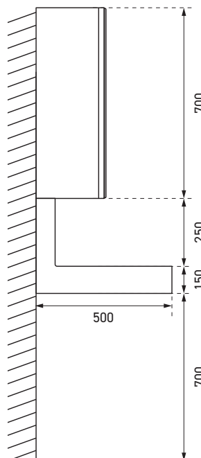
Lavabo matériau composite pour module miroir L600 x H395 x P495 mm REF. LA-600
