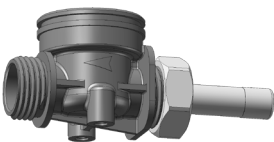
1 X CORPS ÉLECTROVANNE AVEC FILTRE ET RACCORD
