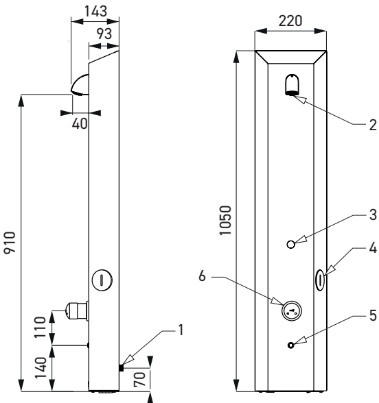
1 - Arrivées eau M1/2" 2 - Pomme de douche 3 - Voyants Leds décompte du temps 4 - Fente introduction jeton 5 - Bouton sensitif Marche/Arrêt 6 - Bouton mélangeur
