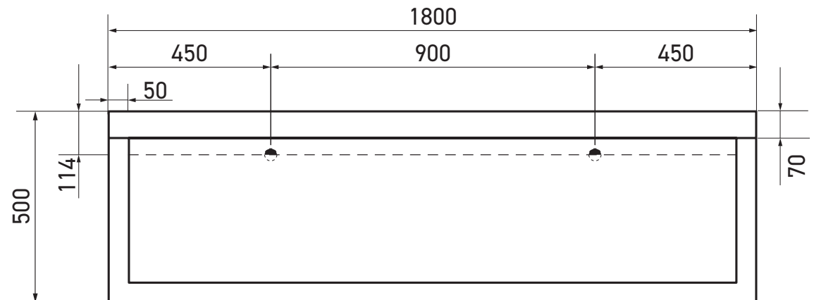
Réf. LVA-1800-D
