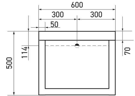
Réf. LVA-600-D
