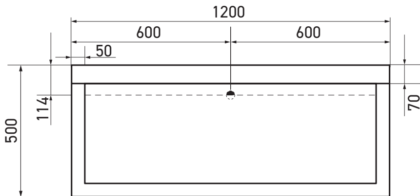
Réf. LVA-1200-D
