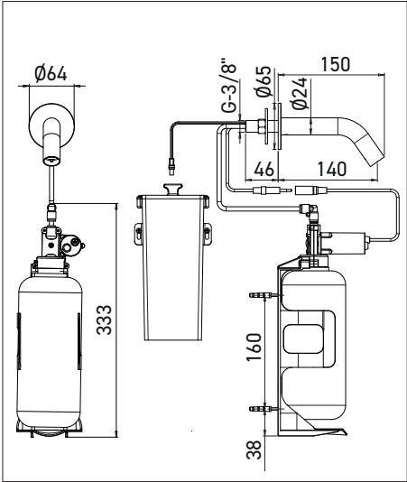
EXTREME WS Réf. RES-641P À piles
