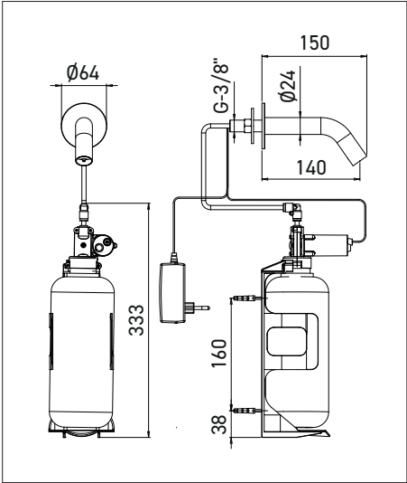
EXTREME WS Réf. RES-641 Sur transformateur
